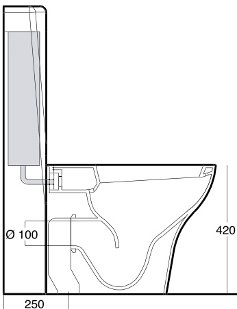
Art. CMBL Cassetta monoblocco completa di batteria di scarico doppio flusso free standing cistern provided with discharge double-flush system
