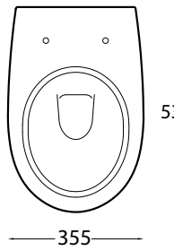
Art. WCESE-001 Vaso Ese sospeso cm.55 Hanging wc bowl Ese cm.55
