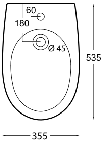
Art. BTSESE-001 Bidet Ese sospeso cm.55 Hanging wc bowl Ese cm.55
