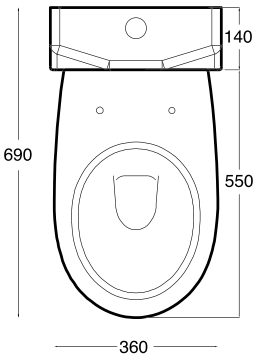
Art. WCESE Vaso a terra Ese cm.55 Ese free standing wc cm.55
