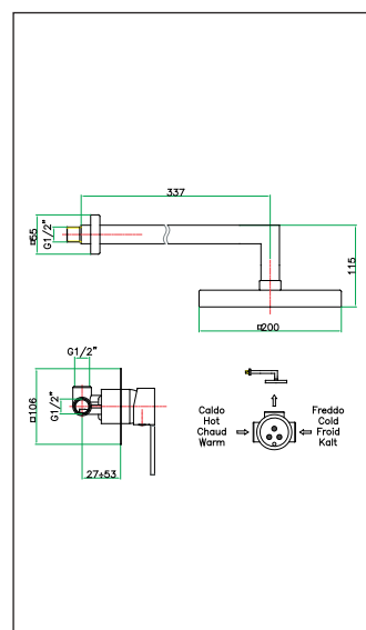
art. 77 CR 7516
