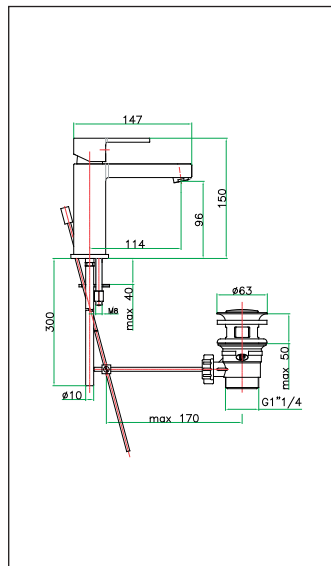
art. 77 CR 7521
