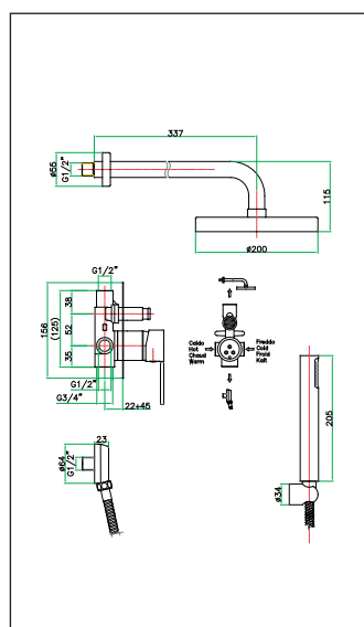
art. 77 CR 7512
