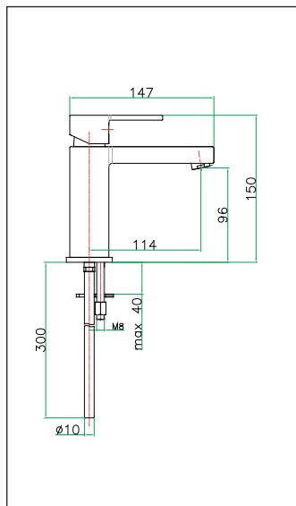
art. 77 CR 7523
