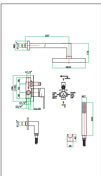
art. 77 CR 7519
