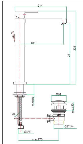
art. 77 CR 7525
