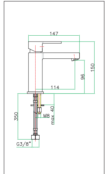
art. 77 CR 7522
