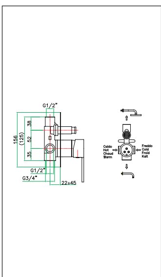
art. 77 CR 7517
