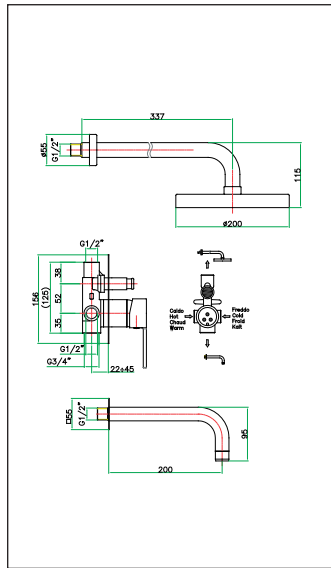
art. 77 CR 7510
