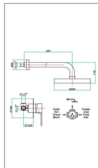
art. 77 CR 7513
