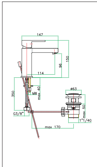
art. 77 CR 7520
