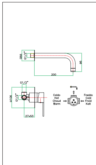
art. 77 CR 7527
