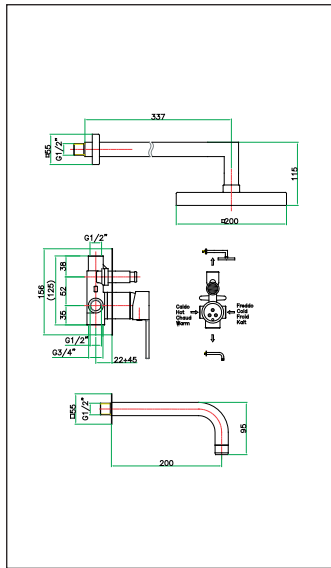
art. 77 CR 7518
