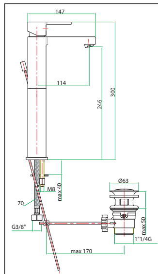
art. 77 CR 7524
