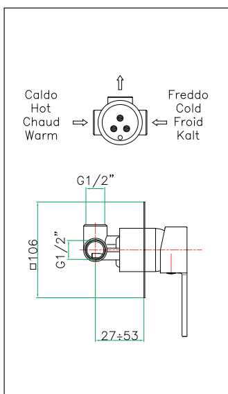
art. 77 CR 7515
