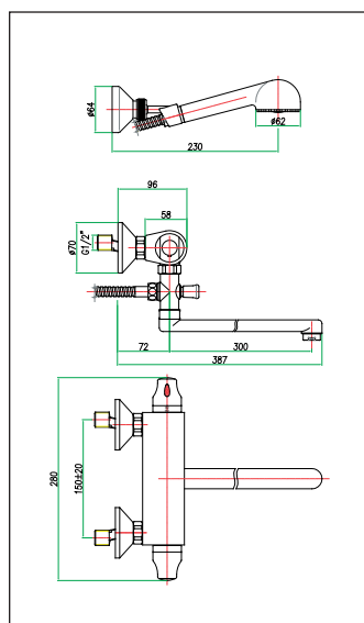
art. 36 CR 0920
