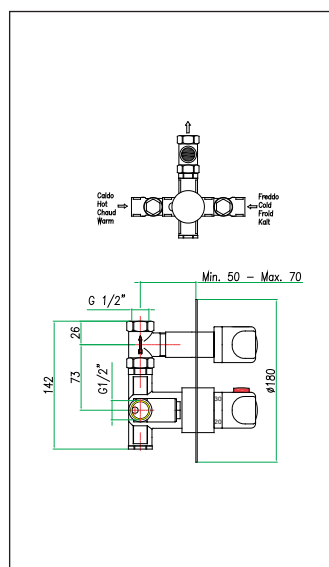
art. 36 CR 0924
