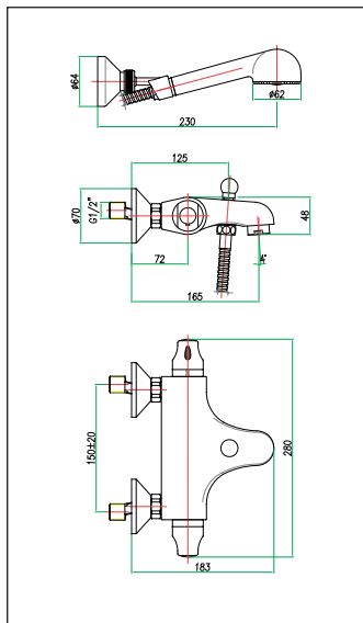
art. 36 CR 0950
