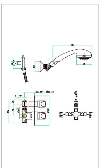
art. 36 CR 0926
