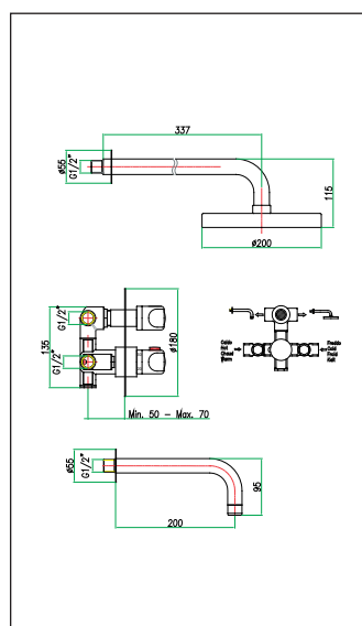
art. 36 CR 0928
