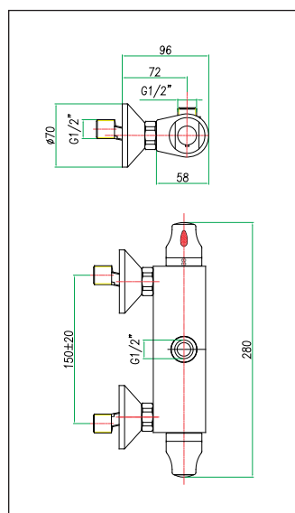
art. 36 CR 0974
