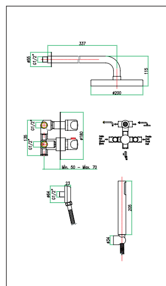
art. 36 CR 0929
