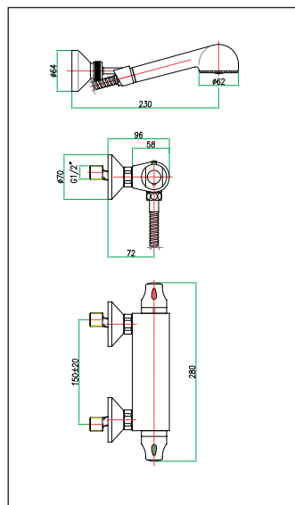
art. 36 CR 0901
