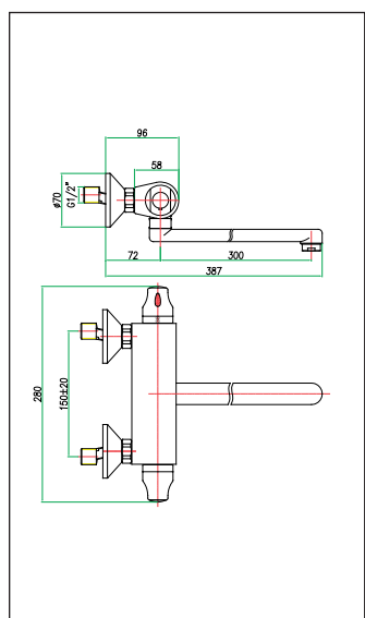
art. 36 CR 0930
