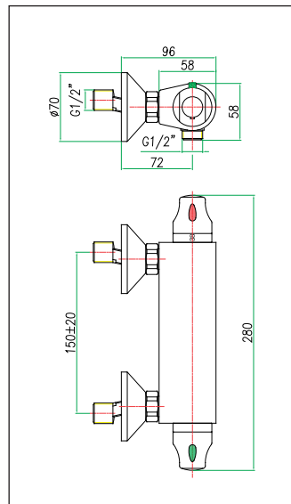
art. 36 CR 0911
