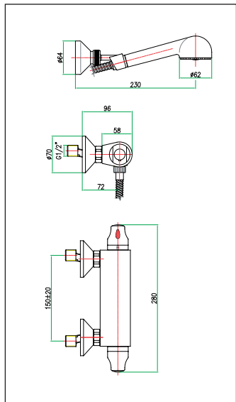
art. 36 CR 0972
