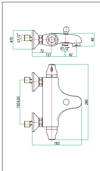
art. 36 CR 0960
