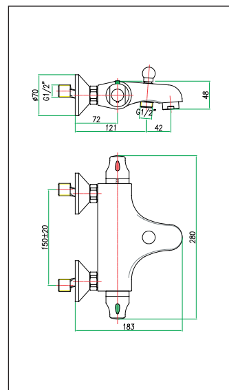
art. 36 CR 0961
