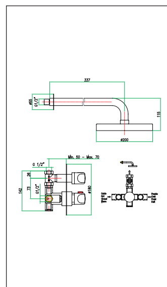
art. 36 CR 0925
