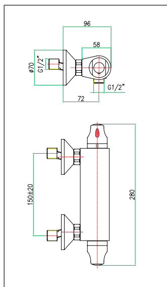
art. 36 CR 0970
