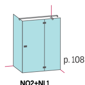
NO2+NL1 porta con segmento fisso in linea e laterale porte avec segment fixe en ligne et latéral door with in-line fixed segment and side panel
