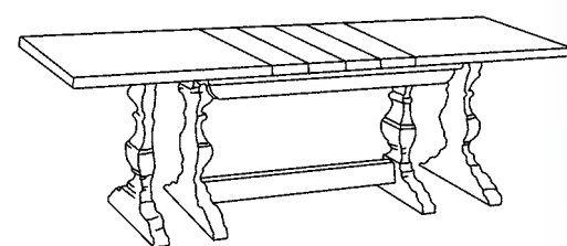
Art. 742/B Tavolo in toulipier riquadrato Extensible table L. 180 P. 85 H. 78 (4 allunghe cm 45 cad.)
