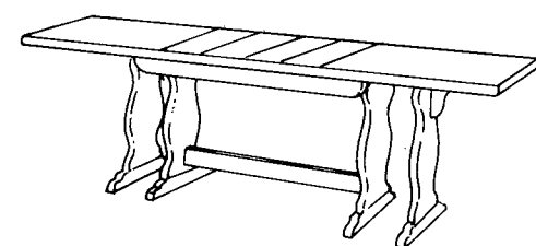
Art. 739/B Tavolo in toulipier riquadrato Extensible table L. 160 P. 85 H. 78 (4 allunghe cm 45 cad.)
