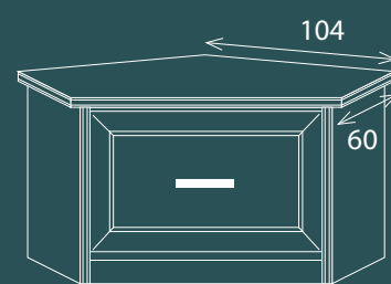
Art. 3043/A Base angolo 1 c. Base cabinet lato 104 P. 115 H. 48
