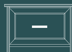
Art. 3040/A Base 1 c. Base cabinet L. 70 P. 60 H. 48
