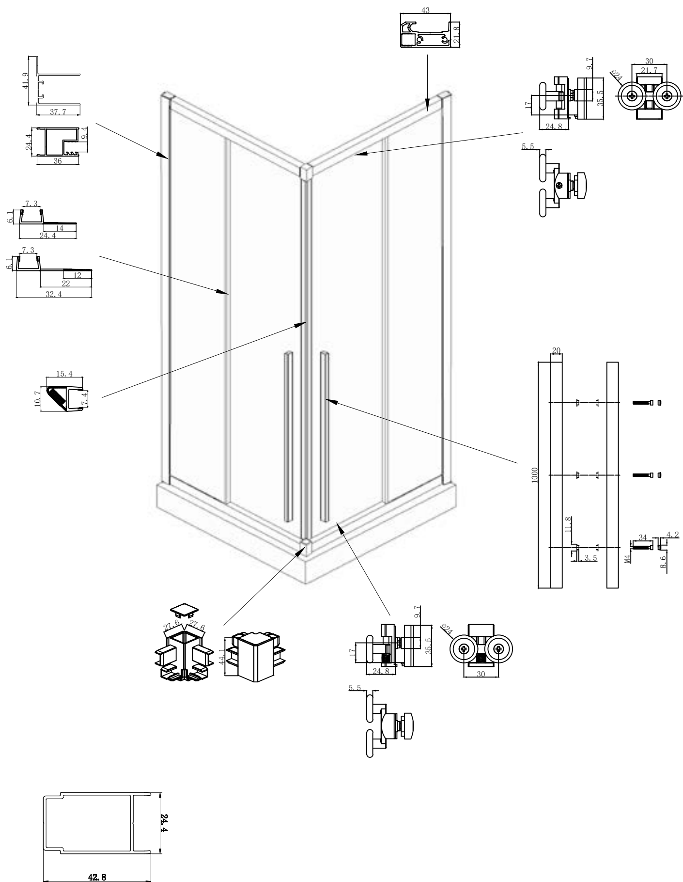
Profilo estensione "11493"
