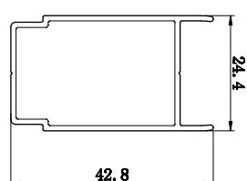
Profilo estensione "11493"
