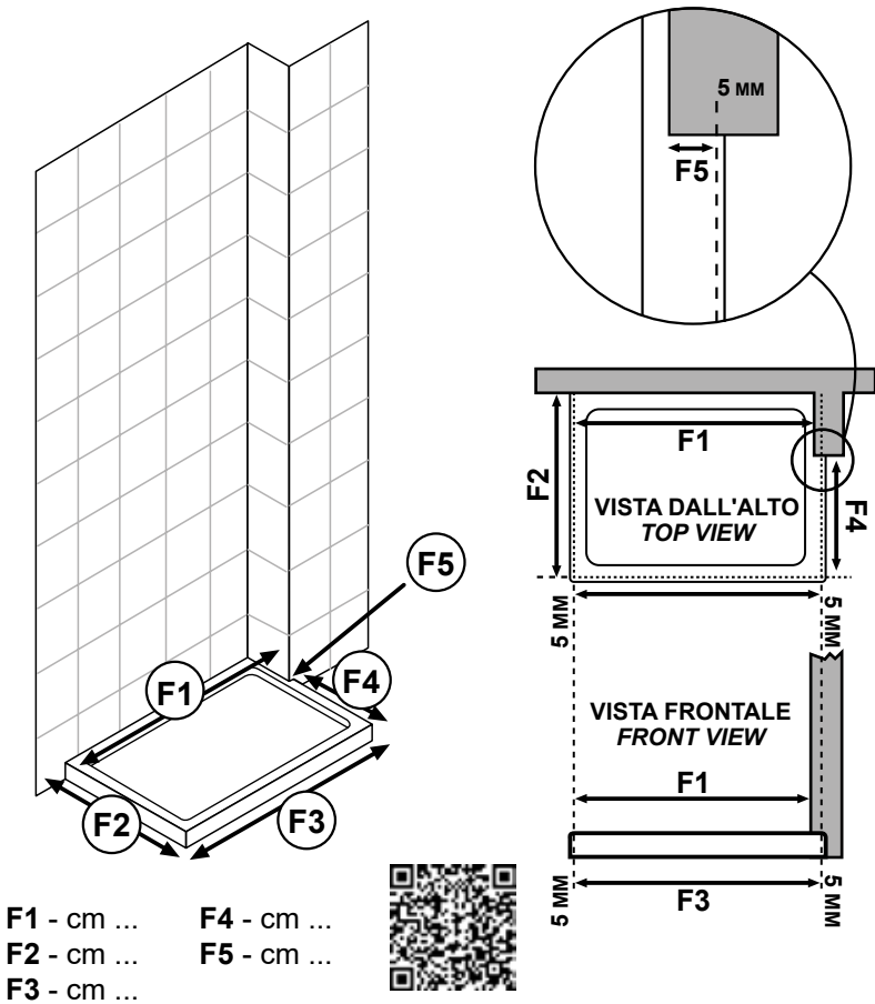
"H" - Spazio in nicchia con muretto Dx Wall-to-wall with low wall to the right. Nische mit niedriger Mauer rechts. Niche avec muret bas à droite.
