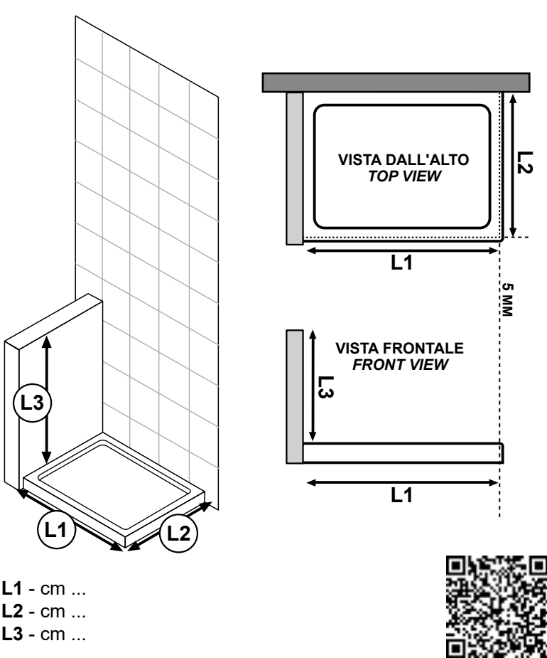
"L" - Spazio in angolo con muretto Sx Corner shower enclosure with low wall to the left. Eck-Duschkabine mit niedriger Mauer links. Cabine de douche en angle avec muret bas à gauche.
