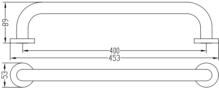
MNGL 45 / 60 Maniglia lineare - Linear handle Linearer Haltgriff - Barre d'appui
