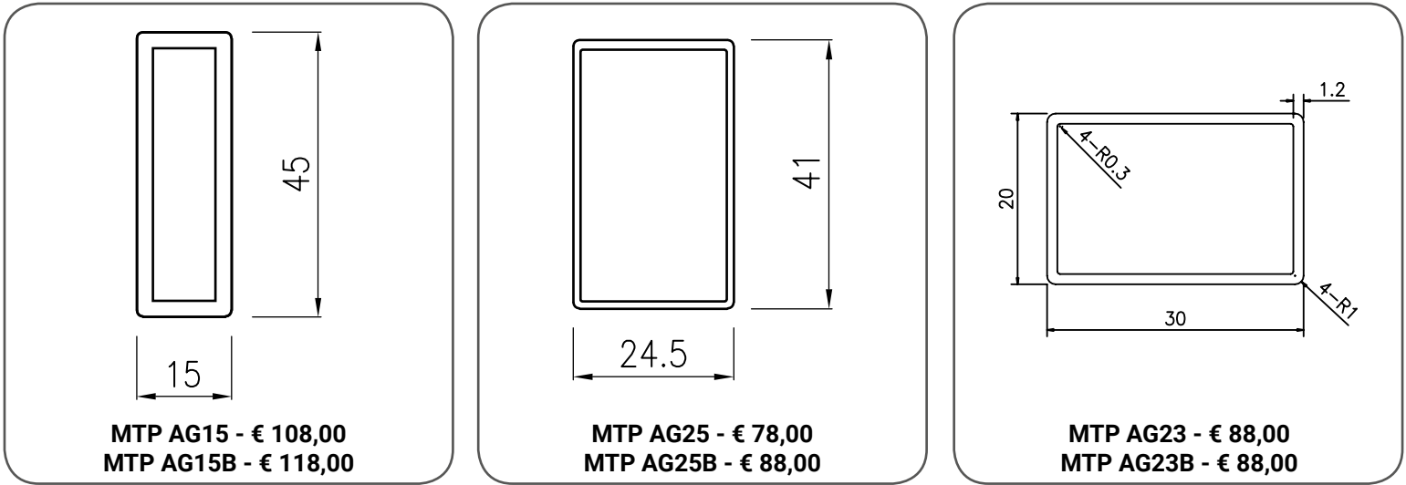
Profili di allungamento in aggiunta. - Additional wall profile adjustment. - Zusätzlicher Verlängerungsprofil. - Profils pour allongement supplémentaire.
