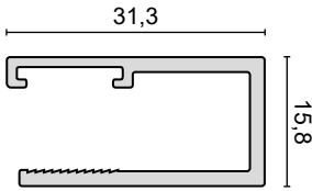
PROFILO A MURO WALL PROFILE - WANDPROFIL - PROFIL DE MUR
