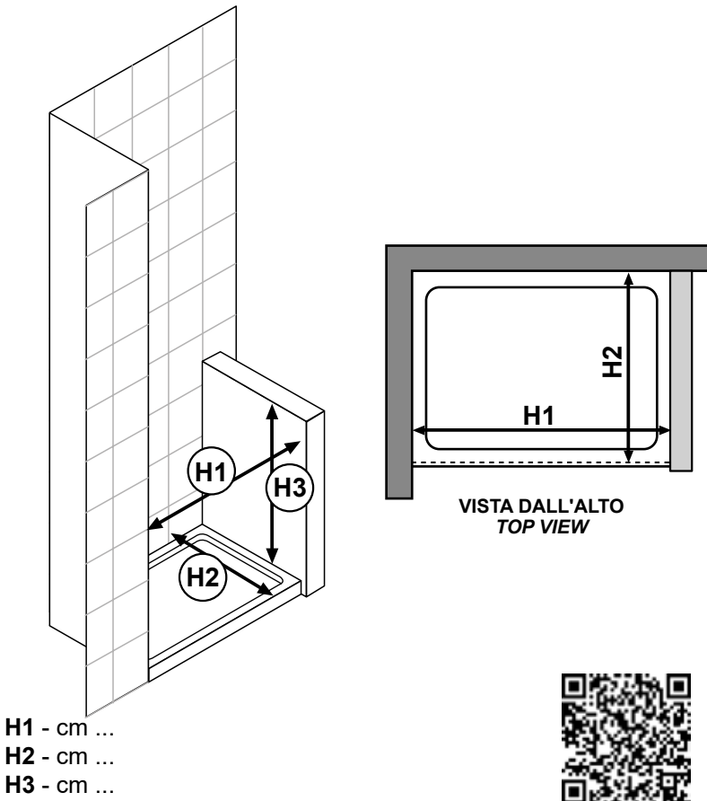
"H" - Spazio in nicchia con muretto Dx Wall-to-wall with low wall to the right. Nische mit niedriger Mauer rechts. Niche avec muret bas à droite.
