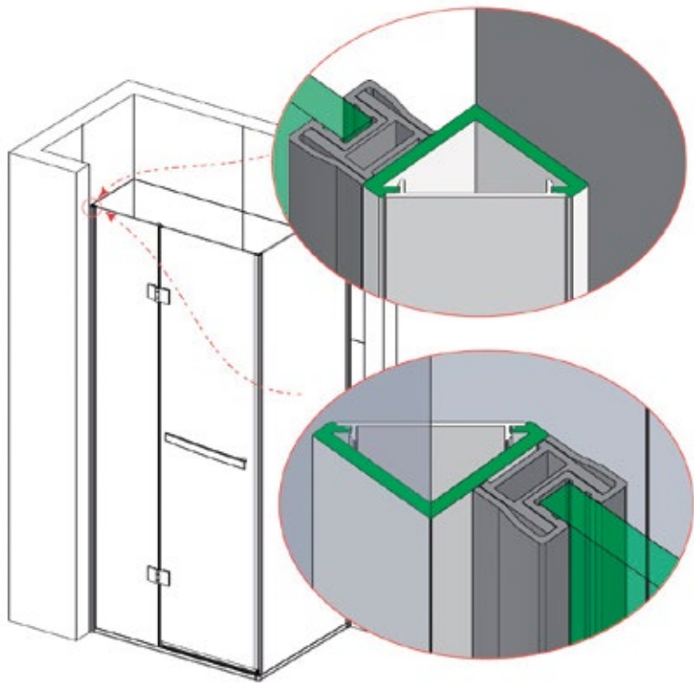
Profilo angolare per fissaggio laterale. Corner profile for lateral fixing. Winkelprofil zur seitlichen Befestigung. Profilé angulaire pour fixation latérale.
