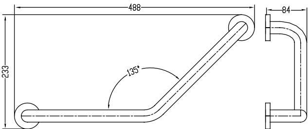
MNGD 45 Maniglia diagonale - Diagonal handle Diagonaler Haltgriff - Barre d'appui coudée
