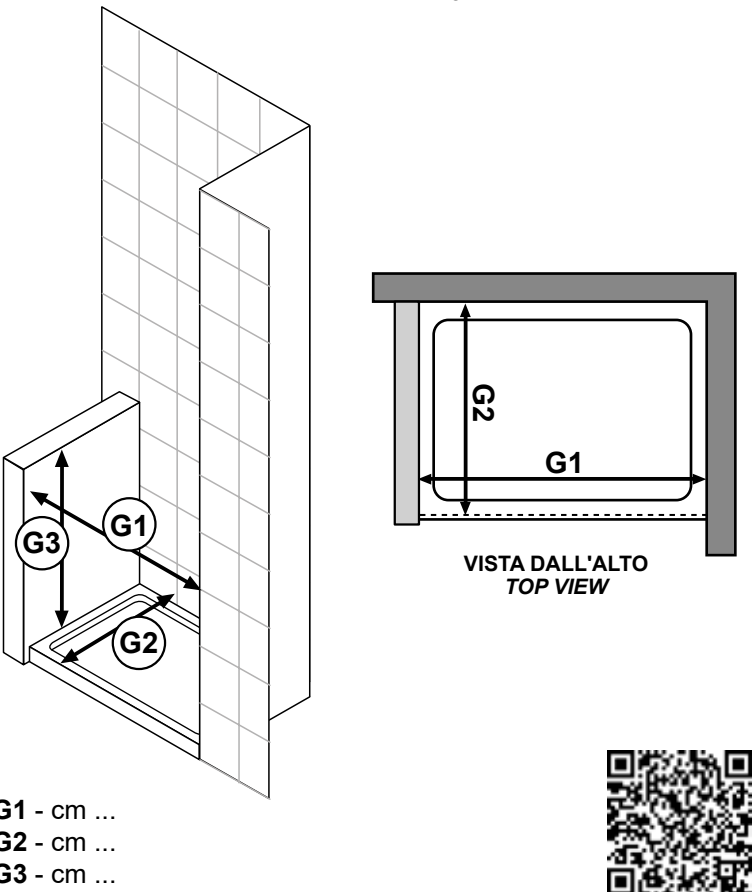
"G" - Spazio in nicchia con muretto Sx Wall-to-wall with low wall to the left. Nische mit niedriger Mauer links. Niche avec muret bas à gauche.
