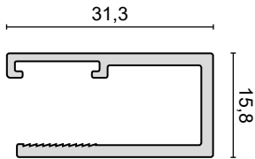
PROFILO A MURO WALL PROFILE - WANDPROFIL - PROFIL DE MUR
