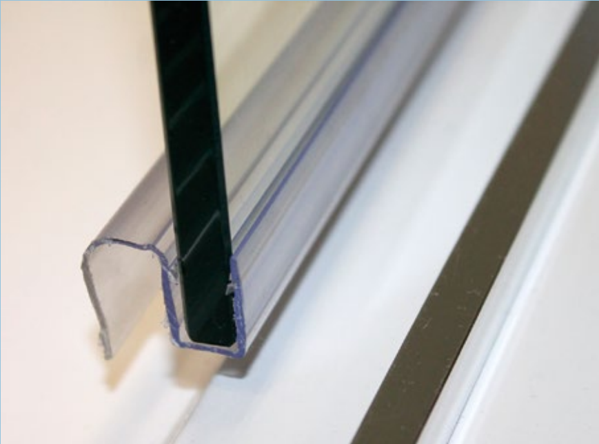
GUARNIZIONE E PROFILO INFERIORE - BOTTOM PROFILE AND GASKET UNTERES PROFIL - JOINT ET PROFILÉ INFÉRIEURE
