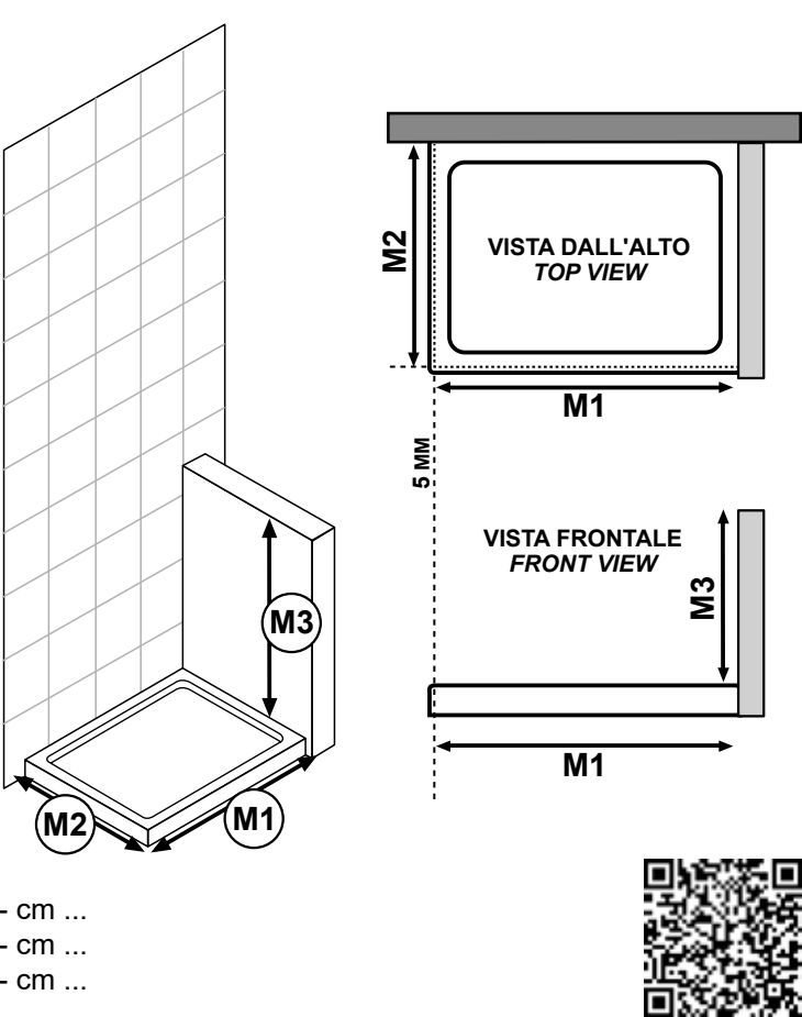
"M" - Spazio in angolo con muretto Dx Corner shower enclosure with low wall to the right. Eck-Duschkabine mit niedriger Mauer rechts. Cabine de douche en angle avec muret bas à droite.
