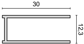
PROFILO A MURO WALL PROFILE - WANDPROFIL - PROFIL DE MUR
