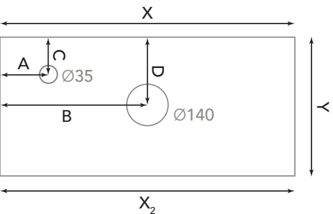
Top con foro per lavabo e rubinetto
