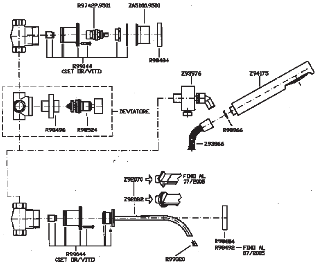
VASCA-DOCCIA ZA5707 Parte esterna External part R99609 Parte incasso con elementi liberi Built-in part not assembled R99617 Parte incasso con corpo unico Assembled built-in part
