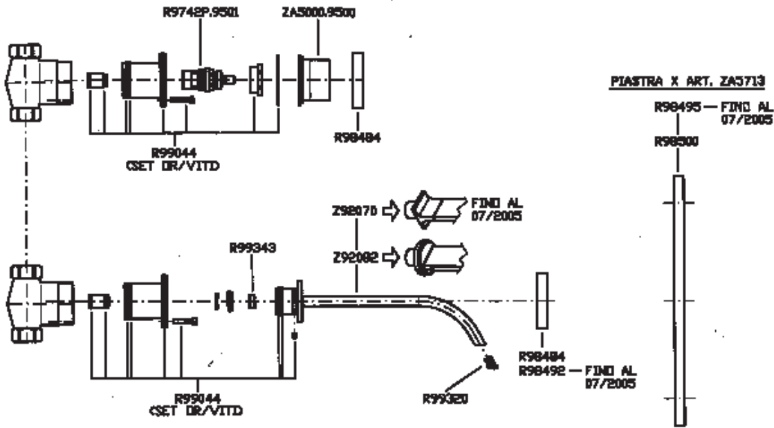
LAVABO ZA5709 Parte esterna External part R99612 Parte incasso con elementi liberi Built-in part not assembled R99615 Parte incasso con corpo unico Assembled built-in part
