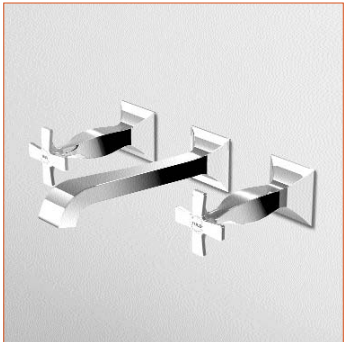
LAVABO ZB1714 Parte esterna External part R99612 Parte incasso con elementi liberi Built-in part not assembled R99615 Parte incasso con corpo unico Assembled built-in part
